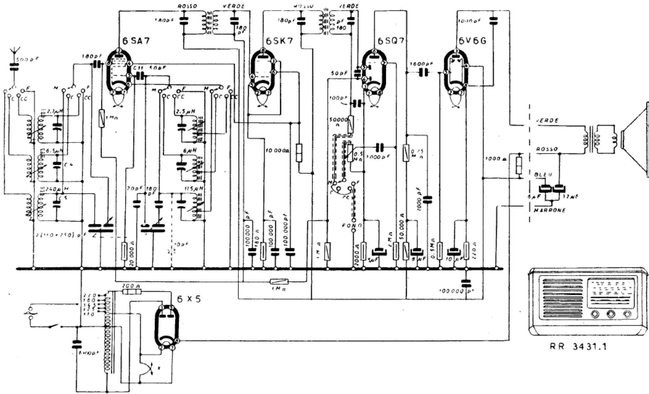
DUCATI - Mod. RR 3431. I Serie METALIST: Gamme onde medie, corte e cortissime. Media frequenza 468 kc. Altoparlante magnetodinamico. Potenza d'uscita 2 W.
